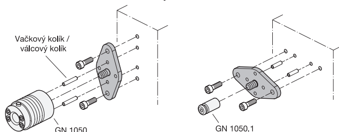
Příklady montáže
