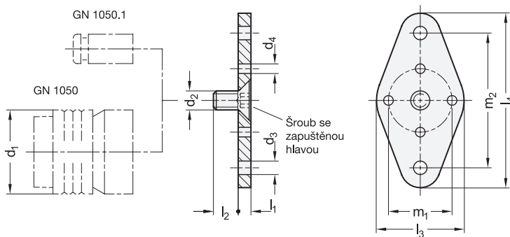
Příklady montáže
